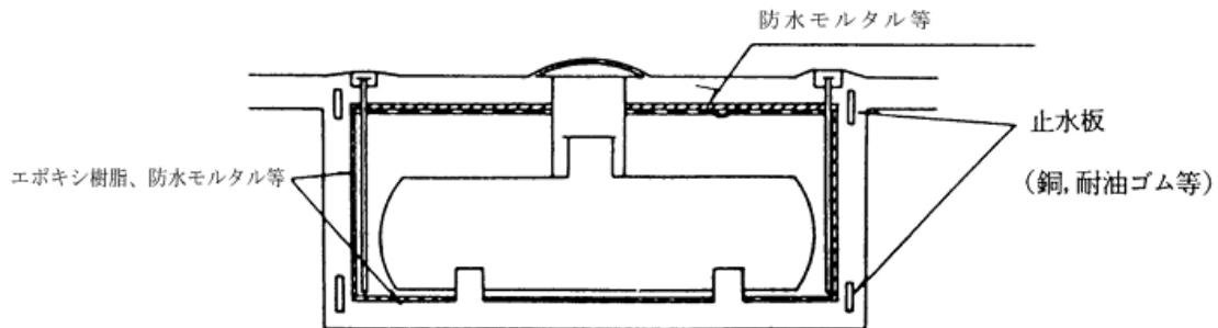
タンク室の防水措置の例
