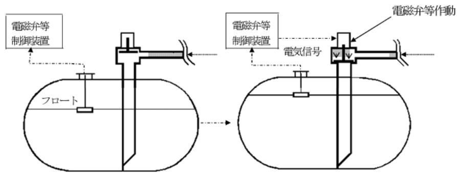
例図3 液面計連動型遮断方式
