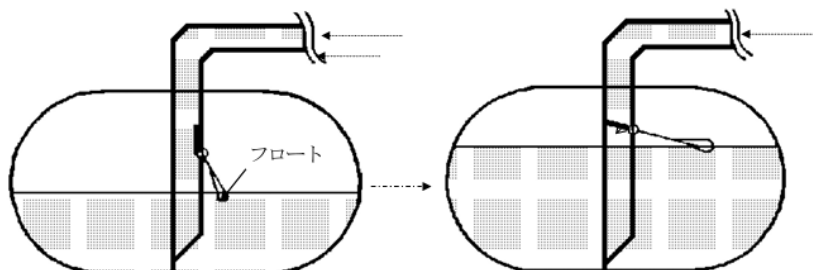
例図2 フロート方式
