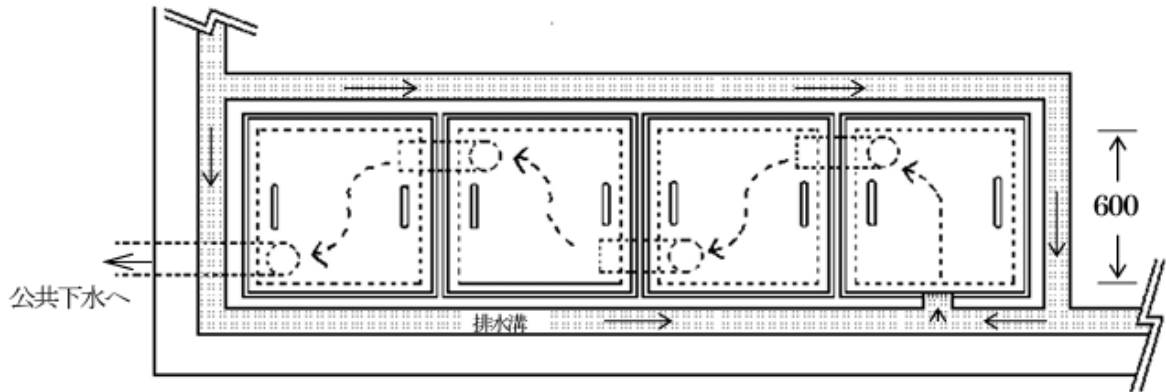
平面図
